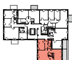
5. OBERGESCHOSS
