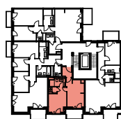
2. OBERGESCHOSS
